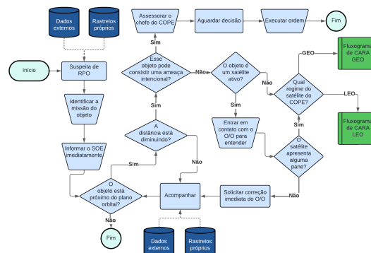
Fig. 7. Fluxograma de atividades para combater suspeita de RPO.
