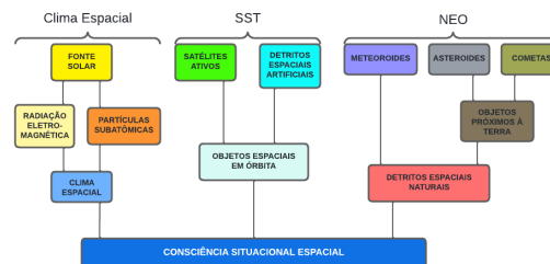
Fig. 2. Componentes relacionados com a SSA. Traduzido de [7].
