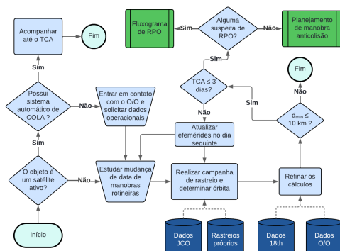
Fig. 5. Fluxograma de atividades para CARA em órbita GEO.
