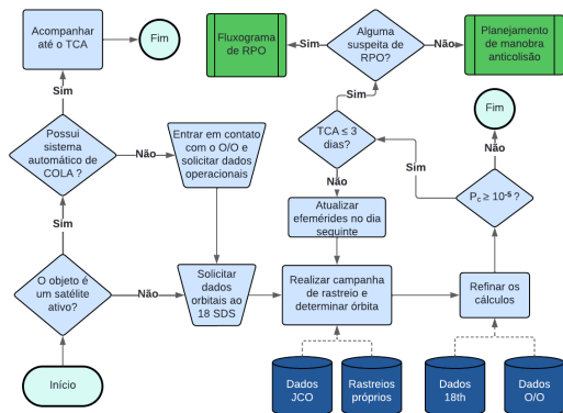
Fig. 4. Fluxograma de atividades para CARA em órbita LEO.
