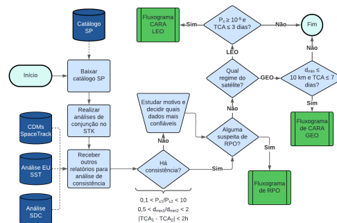
Fig. 3. Fluxograma de atividades para triagem inicial de CA.
