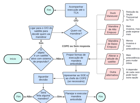
Fig. 6. Fluxograma de planejamento de manobra anticolisão.
